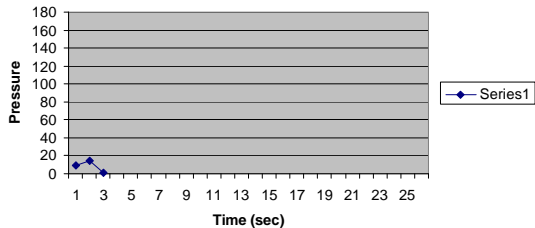
Patient #11 VC (AUC=22)
