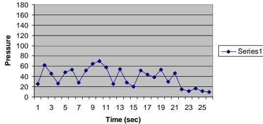
Patient #10 IRCT (AUC=964)
